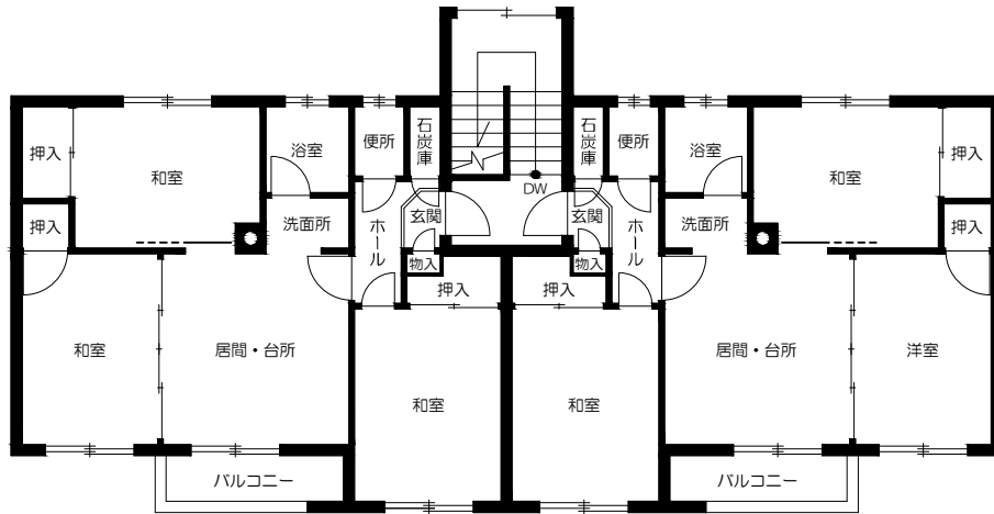
2階平面図
